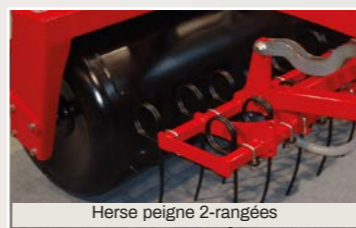
Herse peigne 2-rangées et lame niveleuse
