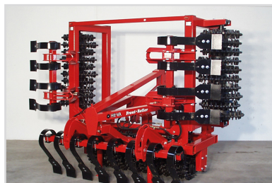
4,00 m Front-Roller m/ Crosskill, hydr. Klappung und Spring-Board.
