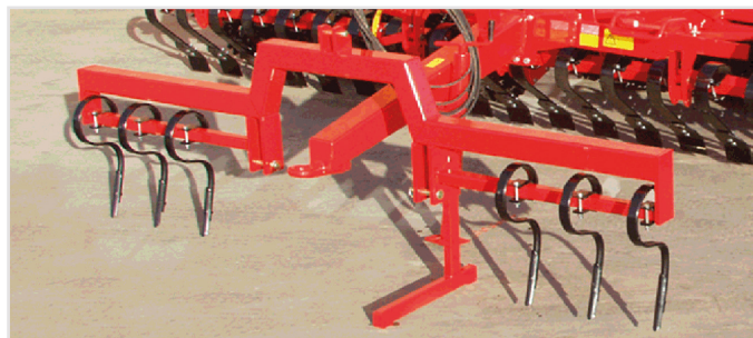
Spårluckringssats, trepunktupphängd
